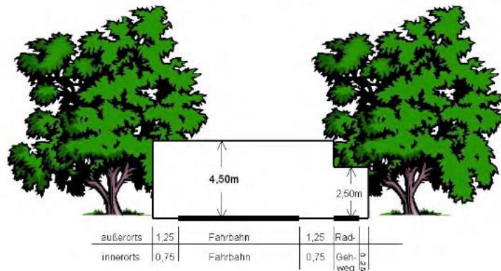
Lichtraumprofil
